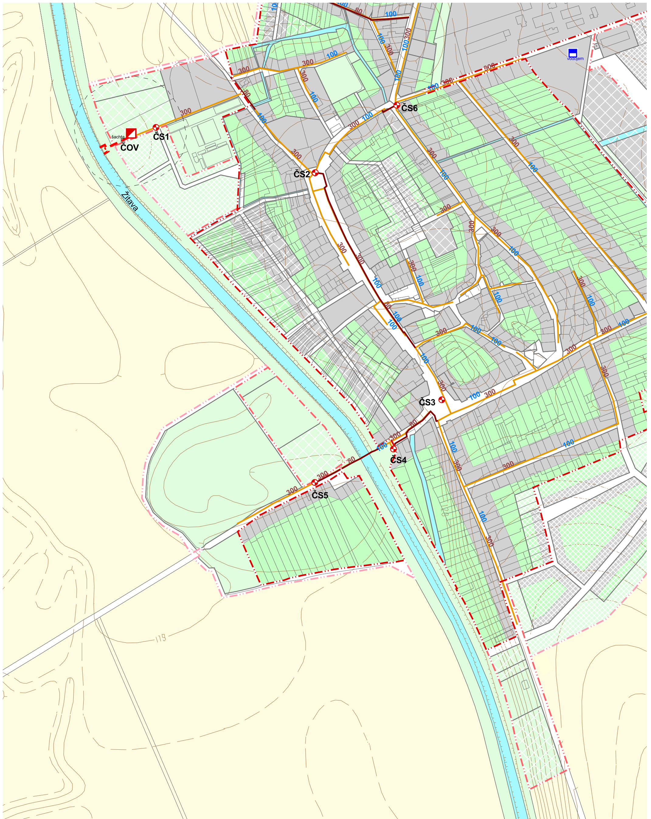
Územný plán obec Bešeňov Zmeny a doplnky č. 2 SÚPN-O Bešeňov - rok 2016 Návrh technickej vybavenosti - voda, kanál 1:5 000 súhrnné znenie 6a
