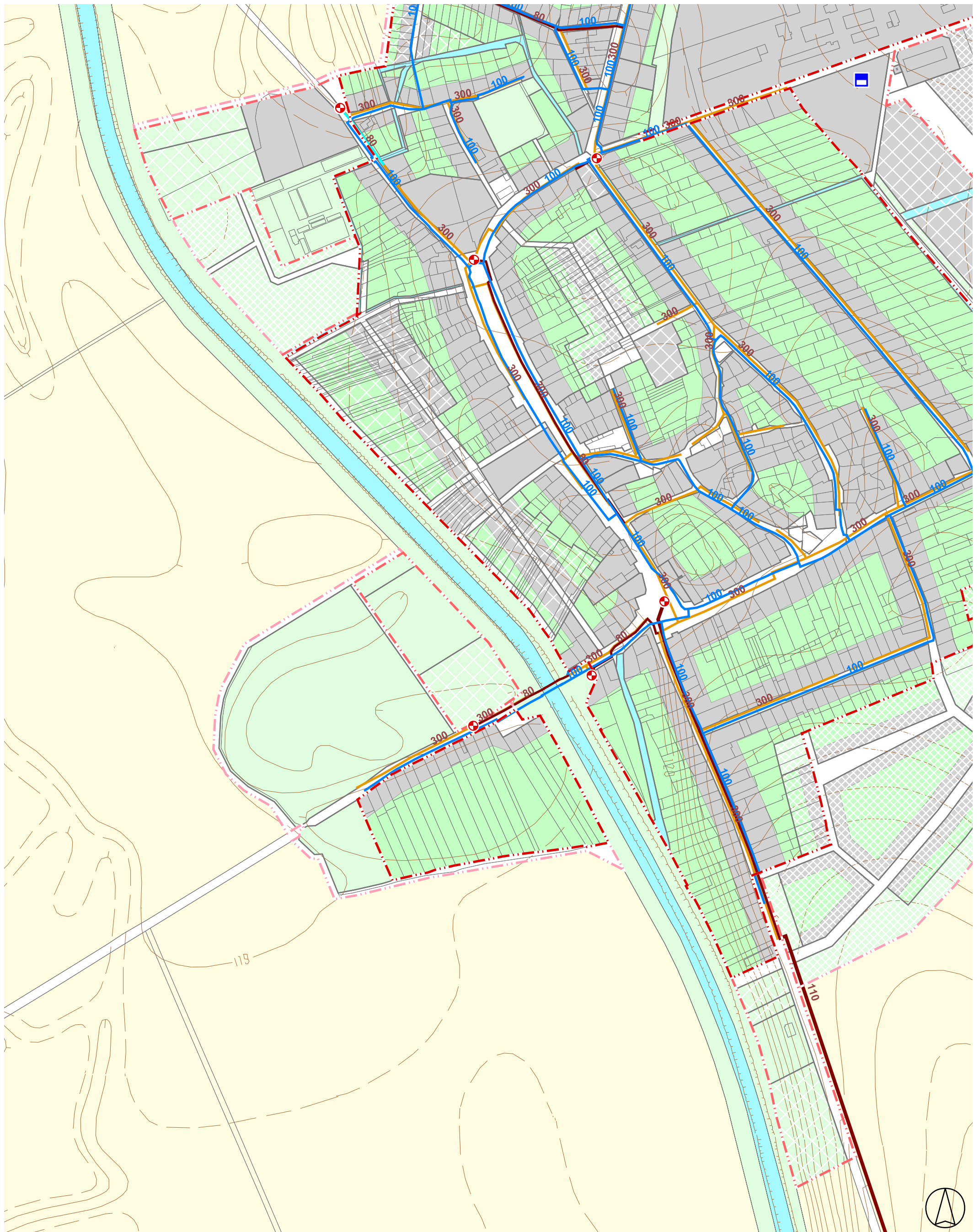
Územný plán obec Bešeňov Zmeny a doplnky č. 2 SÚPN-O Bešeňov - rok 2016 Návrh technickej vybavenosti - voda, kanál 1:5 000 pôvodné znenie 6a
